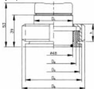
Штуцер 653 / 654
