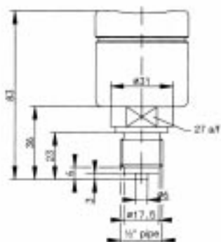
Штуцер 606 / 607
