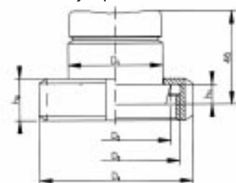
Штуцер 606 / 607
